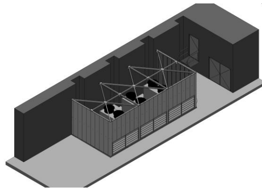
Geluidswand warmtepompen
