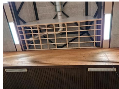
Regelwerk rondom het luchtkanaal
